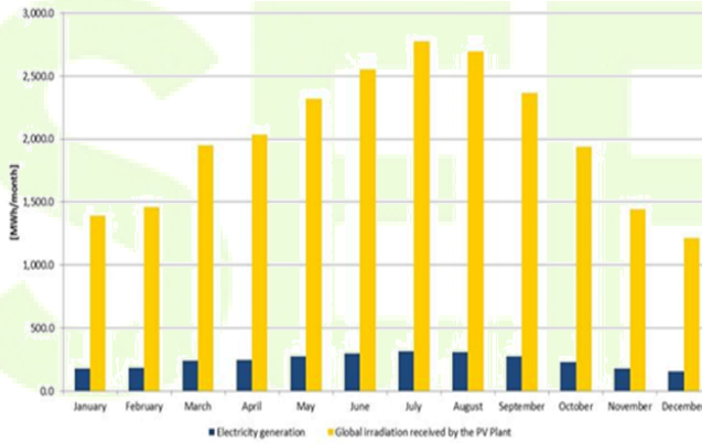
Aylık küresel ışınlama ve elektrik üretimi (1. yıl)
